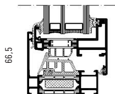
Lodret snit i dreje-kip
