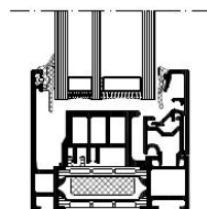
Lodret snit i fast parti
