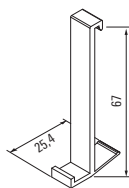
Haken 928 164 Hook 928 164
