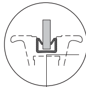
Füllungseinfassprofil 552 637 für 4 mm Stärke 552 647 für 6 mm Stärke 552 657 für 8 mm Stärke Infill frame edge profile 552 637 for 4 mm thickness 552 647 for 6 mm thickness 552 657 for 8 mm thickness
