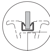
Füllungseinfassprofil 552 637 für 4 mm Stärke 552 647 für 6 mm Stärke 552 657 für 8 mm Stärke Infill frame edge profile 552 637 for 4 mm thickness 552 647 for 6 mm thickness 552 657 for 8 mm thickness
