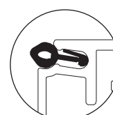
Staubdichtung 650 058 für Profil 923 088 Dust-repellent gasket 650 058 for profile 923 088
