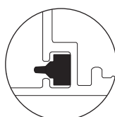
Dichtung 650 010 für Profil 923 150 Gasket 650 010 for profile 923 150
