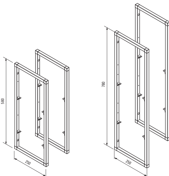
Set Seitenteil 580 mm 928 515 Kit for 580 mm side component 928 515
