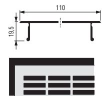
Art.-Nr. 921 541 rechteckig, 30 x 5,7 mm Lüftungsquerschnitt: 496 cm 2 /m Art. No. 921 541 rectangular, 30 x 5.7 mm Ventilation cross-section: 496 cm 2 /m
