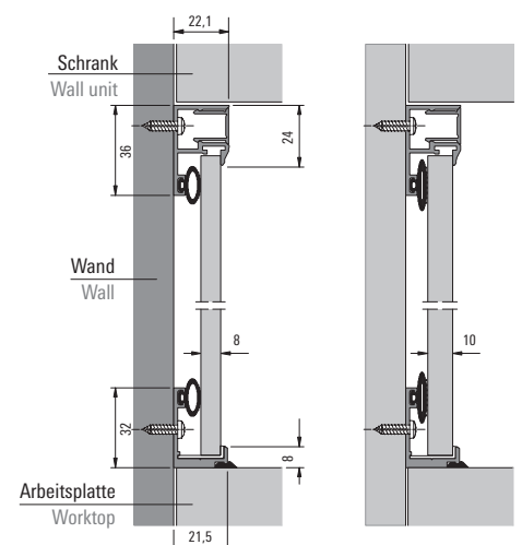
Nischenmontage Midway installation (Beispiel 8 mm) (Beispiel 10 mm) (Example 8 mm) (Example 10 mm)
