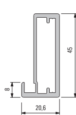
Profil 901 070 Profile 901 070
