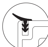
Feuchtigkeitsdichtung 532 837 für Profil 923 087 Moisture-repellent gasket 532 837 for profile 923 087
