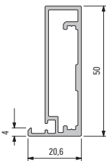
Profil 923 150 Profile 923 150
