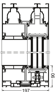
Vertikální řez Schüco ASS 77 PD.HI, měřítko 1:8 Vertical section detail Schüco ASS 77 PD.HI, scale 1:8
