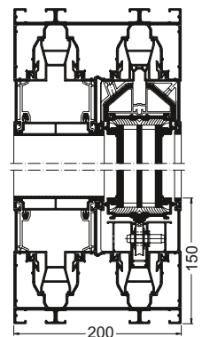
Vertikální řez Schüco ASS 77 PD.NI, měřítko 1:8 Vertical section detail Schüco ASS 77 PD.NI, scale 1:8
