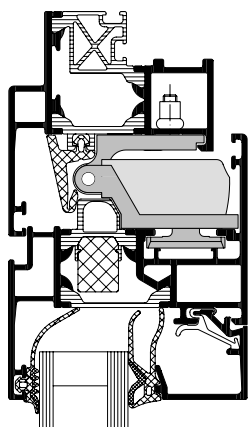
Horizontale doorsnede Schüco TipTronic SimplySmart
