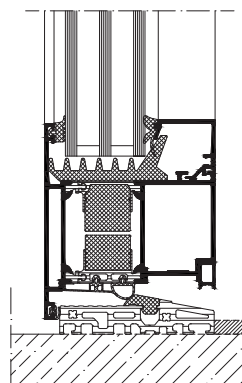
Anslutningsprincip, skala 1:4
