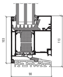
Profilmått, skala 1:4
