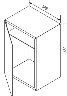
Box mit Tür 928 432 Box with door 928 432
