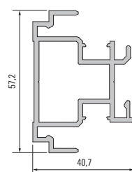
Grundträger 928 160 Base support 928 160
