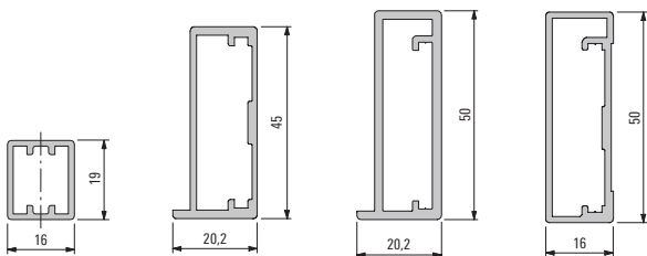
Profil 923 062 Profile 923 062
