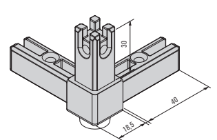
Eckknoten 3s mit Stellfuß 565 386 Corner joint, 3-sided, with adjustable foot 565 386
