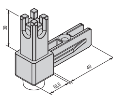
Eckknoten 2s mit Stellfuß 565 406 Corner joint, 2-sided, with adjustable foot 565 406
