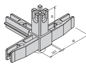
Eckknoten 4sh mit Stellfuß 565 396 Corner joint, 4-sided, horizontal with adjustable foot 565 396
