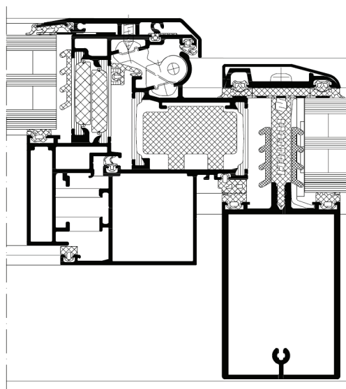
profilsnitt
