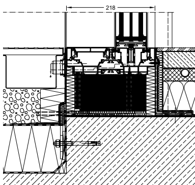
Eksempel på bunndetalj: Access Line
