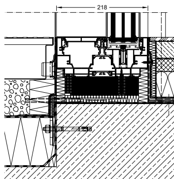
Eksempel på bunndetalj: Design Line
