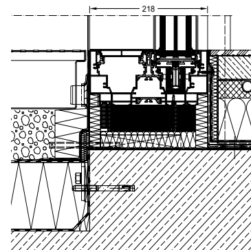
Eksempel på bunndetalj: Performance Line
