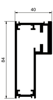
Profilé de porte premium L-XL Profilo porta Premium L-XL
