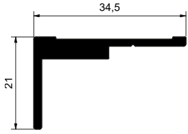
Profilé de logement de panneau technique Profilo di montaggio pannello tecnico
