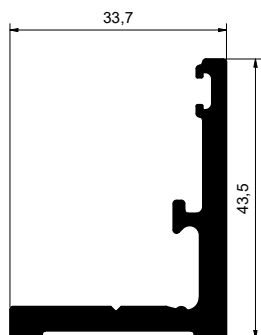
Profilé de base Profilo base
