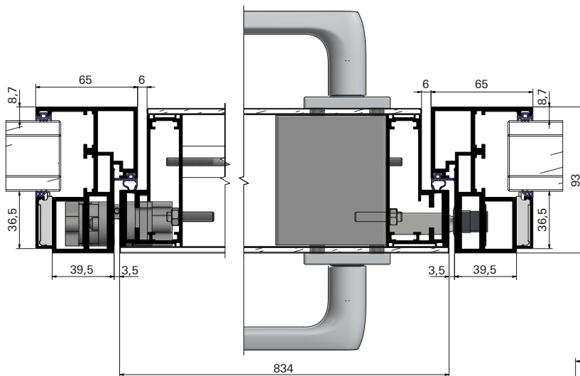
Coupe horizontale DIN gauche Sezione orizzontale DIN sinistro
