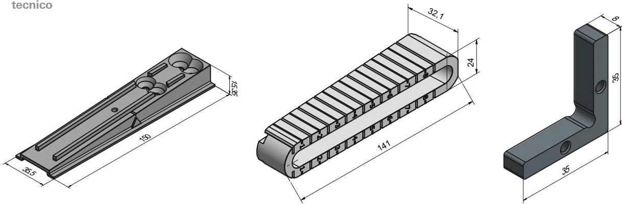
Support de vitrage pour panneau technique de support Supporto a binario per pannello tecnico portante
