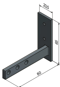
Équerre de fixation au sol de profilé de châssis Staffa a pavimento profilo per controtelaio
