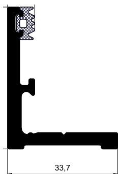
Profilé de base avec joint de base intégré Profilo base con guarnizione base retratta
