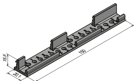
Clip de parclose de châssis de base S Bloccaggio per fermavetro controtelaio di base S
