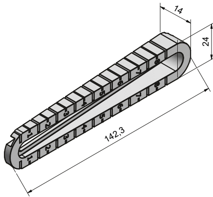
Glissière pour panneau technique de support S Slitta per pannello tecnico portante S
