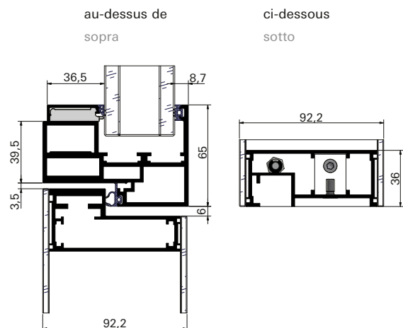
Coupe horizontale en haut/en bas Sezione orizzontale in alto/in basso
