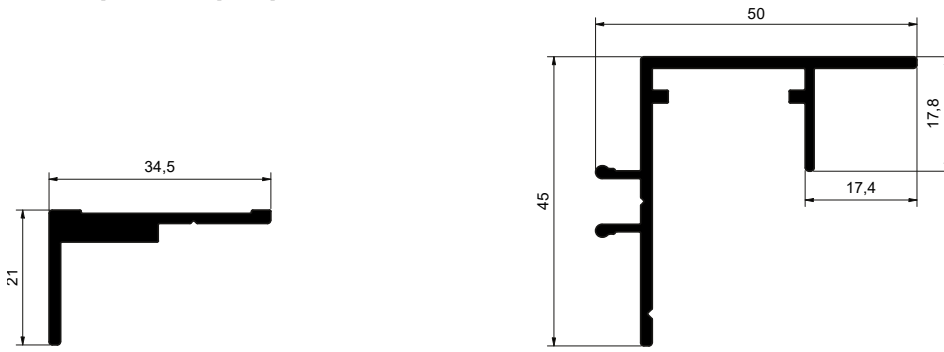
Profilé de logement de panneau technique Profilo di montaggio pannello tecnico
