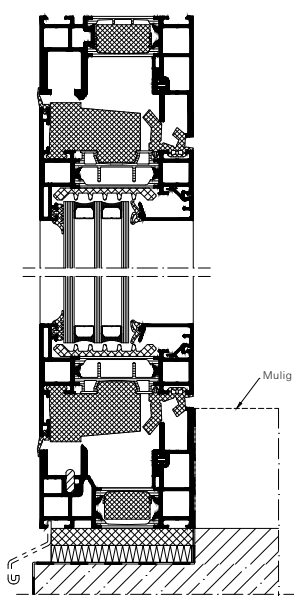
Tilslutningsprinsipp foldesystem
