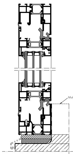
Tilslutningsprinsipp foldesystem
