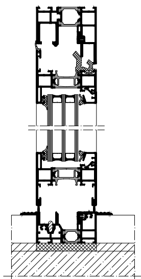
Detalj med nedsenket terskel
