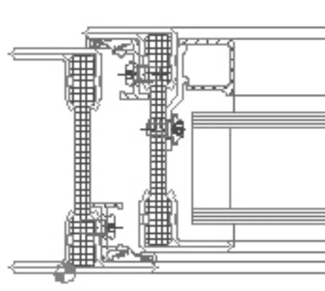
Ramme med karm på 40 mm profilbredde
