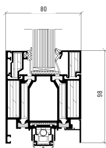
Profilmål, skala 1:4
