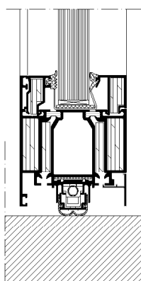
Bunndetalj heveterskel, skala 1:4
