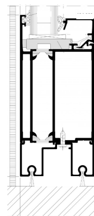
Bunnsnitt automatikkfelt
