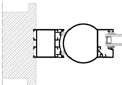
Tilslutningsprinsipp med klemfri bakkant
