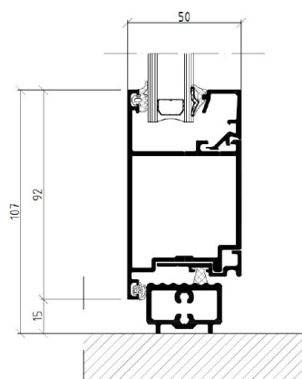
Profilmål terskelløsning
