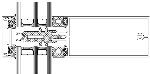
Vertikalsnitt
