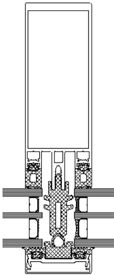
Horizontalsnitt
