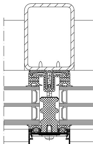
Horizontalsnitt
