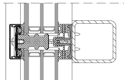
Vertikalsnitt
