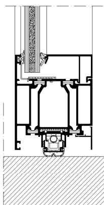
Bunndetalj heveterskel, skala 1:4
