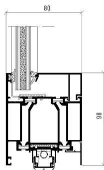
Profil mål, skala 1:4
