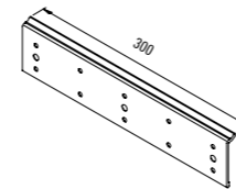
928 091.73.99 Listón de montaje 300 mm con saliente de fijación
