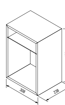
928 411 Box, abierto
