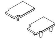
530 017 Tapas de remate izquierda 530 027 Tapas de remate derecha
