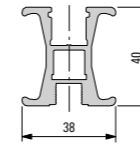
928 036 Perfil de maneta C
