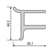
902 181 Perfil portante para suelos 16 mm
