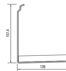
928 431 Anaquel
