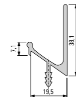
901 231 Perfil
