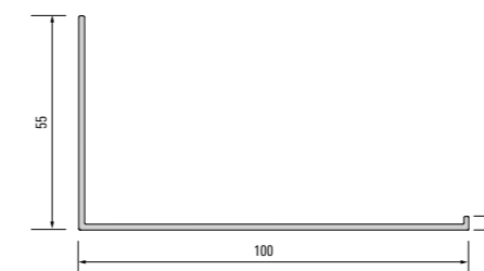
928 115 Perfil de separación
