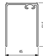
928 061 Carril guía, de una rodadura
