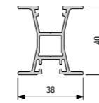
928 102 Perfil de maneta C Basic
