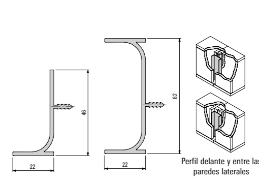
901 009 Perfil 901 010 Perfil
