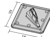
565 466 Alojamiento
