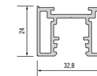
928 183 Maneta
