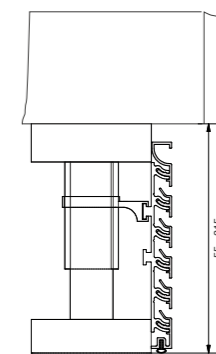
Sección transversal de ventilación: 54-490 cm 2 /m
