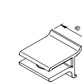
902 625.61.99 Soporte para fondos de vidrio 8 mm
