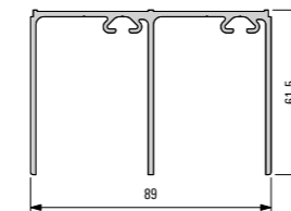
928 060 Carril guía, de dos rodaduras
