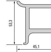
903 011 Perfil portante de suelo 25 mm
