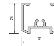
928 186 Marco superior / inferior
