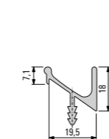
901 232 Perfil
