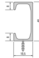
901 052 Perfil Reta
