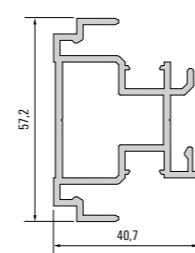
928 160 Soporte básico
