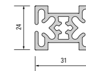
928 188 Parteluz
