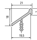
901 108 Perfil Ladeo
