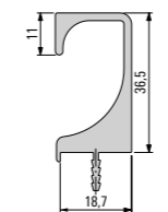
900 303 Perfil
