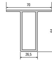
911 053 Traviesa central
