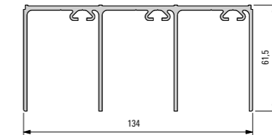
928 051 Carril guía, de tres rodaduras
