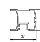
928 095 Perfil de maneta cepillo BAL
