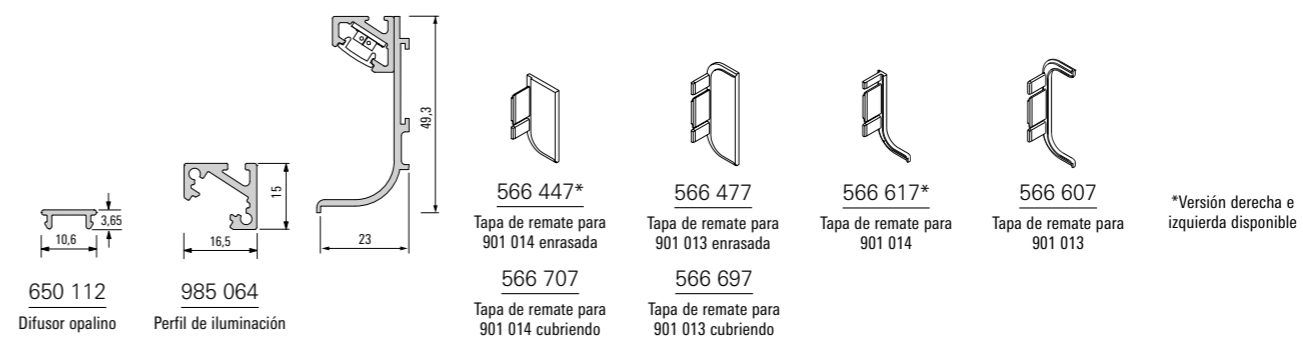
650 112 Difusor opalino 985 064 Perfil de iluminación 566 447* Tapa de remate para 901 014 enrasada 566 477 Tapa de remate para 901 013 enrasada 566 617* Tapa de remate para 901 014 566 607 Tapa de remate para 901 013 566 707 Tapa de remate para 901 014 cubriendo 566 697 Tapa de remate para 901 013 cubriendo
