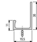
901 246 Perfil
