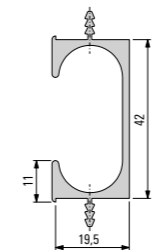
900 452 Perfil
