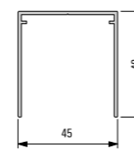
928 097 Carril guía, de una rodadura
