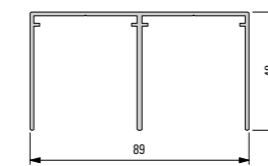
928 094 Carril guía, de dos rodaduras
