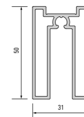
928 187 Marco inferior herraje de ruedas
