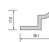
928 185 Listón de montaje
