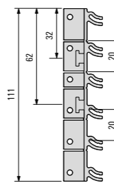
530 087 Alojamiento de fijaciones de material sintético derecha/izquierda
