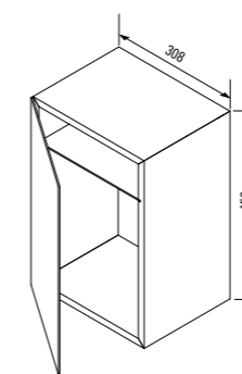
928 432 Box con puerta
