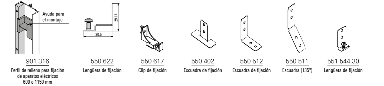
901 316 Perfil de relleno para fijación de aparatos eléctricos 600 o 1150 mm 550 622 Lengüeta de fijación 550 617 Clip de fijación 550 402 Escuadra de fijación 550 512 Escuadra de fijación 550 511 Escuadra (135°) 551 544.30 Lengüeta de fijación
