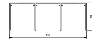
928 096 Carril guía, de tres rodaduras
