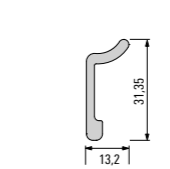
902 150 Perfil de montaje para pernos de estante
