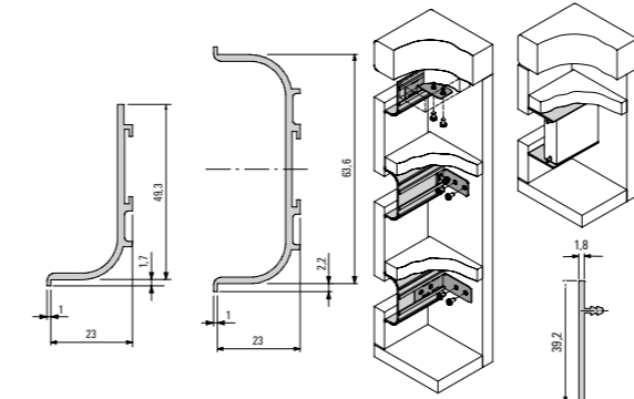
901 014 Perfil 901 013 Perfil 901 053 Perfil
