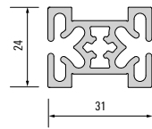
008687 Bar
