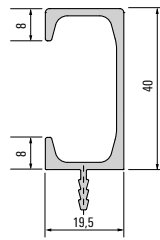
004457 Reta profile
