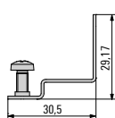
550 622 Fixing lug
