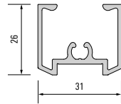
008677 Frame, top / bottom
