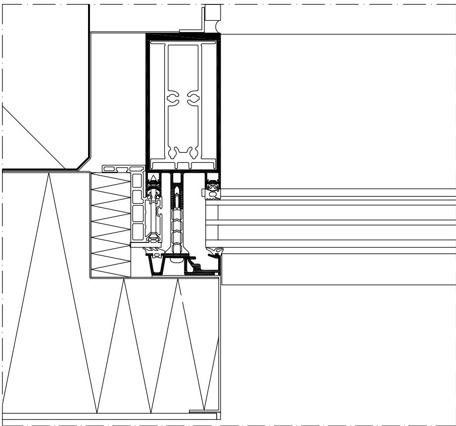
Bouwkundige aansluiting FWS 35 PD
