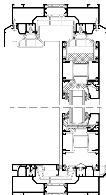
Vertikalt snitt
