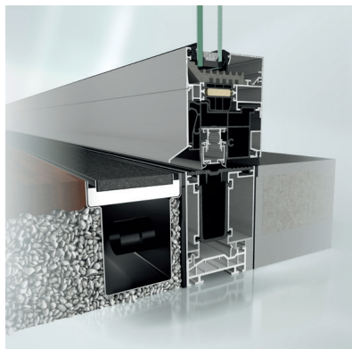
AWS 75.SI+ med barrierefri nullnivå-terskel
