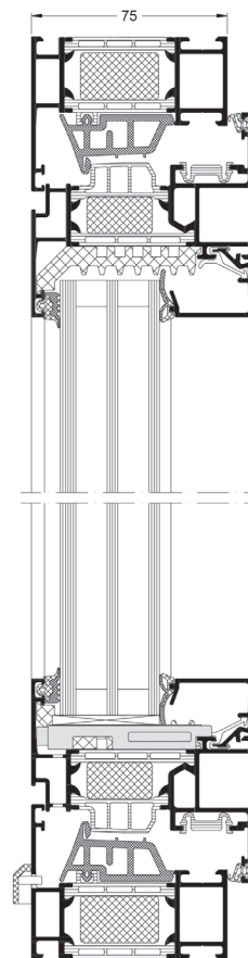
AWS 75.SI+ vertikalt snitt 1:2
