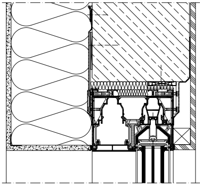
Tilslutningsprinsipp overkant dør
