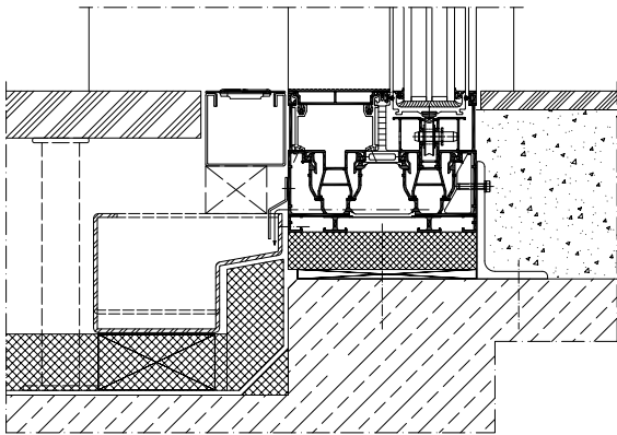
Tilslutningsprinsipp gulv
