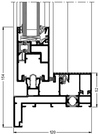
Baseprofil for høyere slagregntetthet
