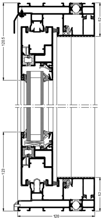
Vertikalsnitt 1-spors dør målestokk 1:2
