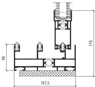
3-spors skyveparti
