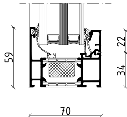
Vertikalsnitt gjennom fastkarm, målestokk 1:2
