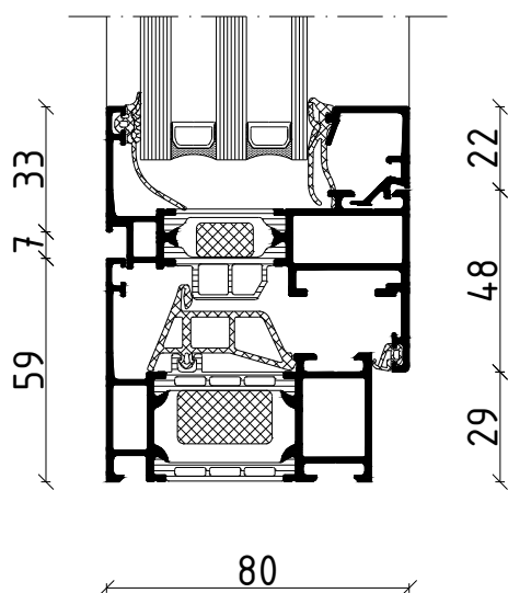
Vertikalsnitt gjennom åpningsvindu, målestokk 1:2
