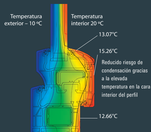
Corona CT 70 Termografía de la sección
